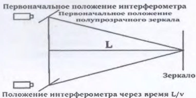
Рис. 2. Схема движения света в опыте Майкельсона, направленного перпендикулярно к движению Земли
